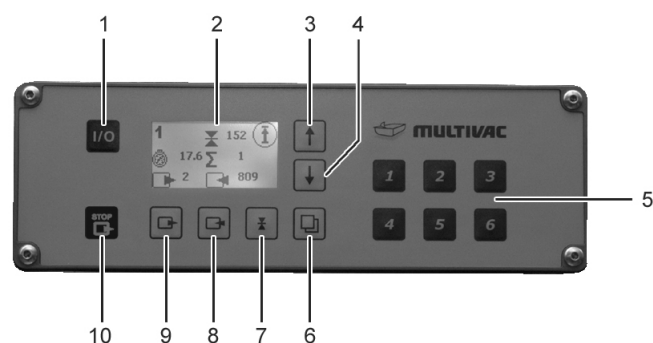
Рис. 4: Пульт управления
