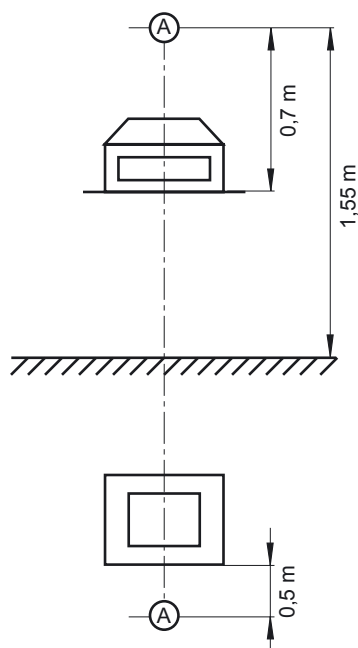
Рис. 8: Точка измерения уровня шума
