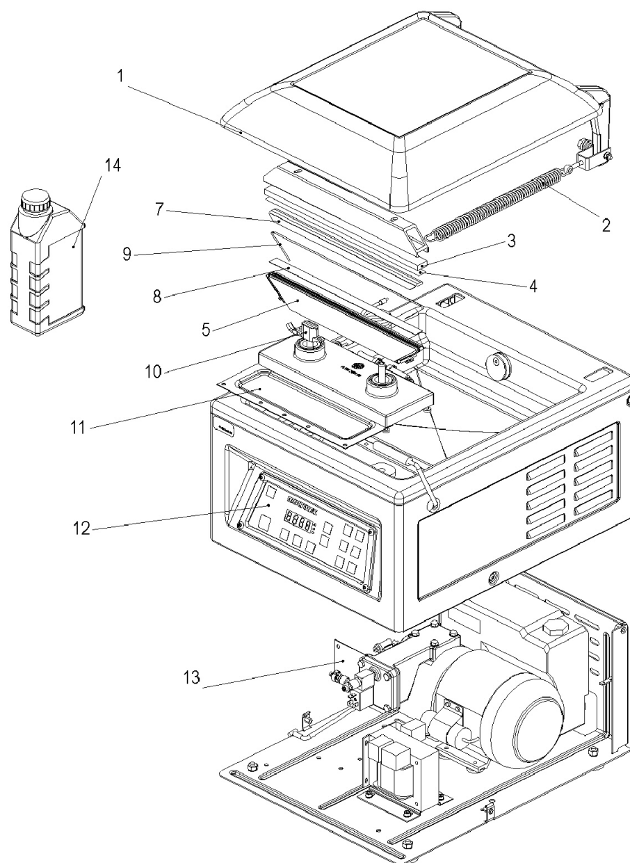
Рис. 10: Чертеж запасных частей (SAP-DIS 16000015492)
