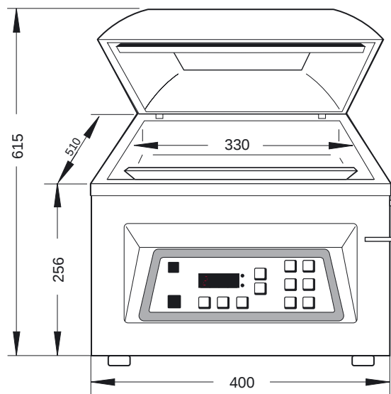
Рис. 7: Размеры
